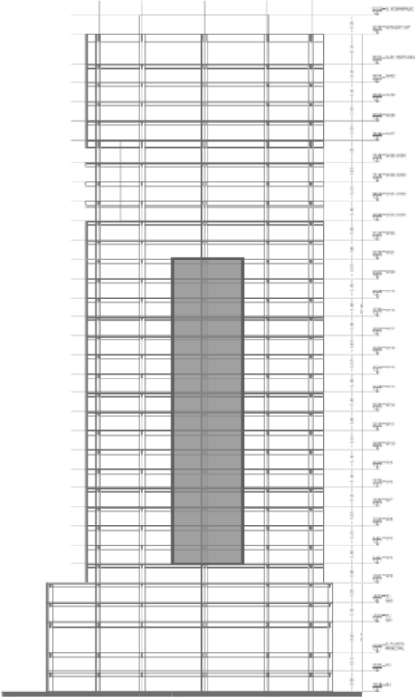
SECCIÓN DE REFERENCIA
